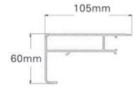
Profil oben/unten
