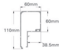
Profil links/rechts
